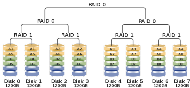
Figura 9: RAID 1+0+0.
