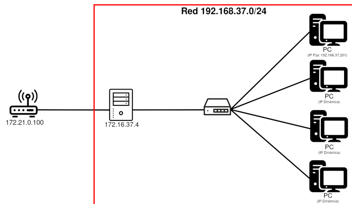
Figura 2: Diagrama de nuestra red.
