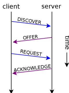
Figura 1: Diagrama del protocolo DHCP.
